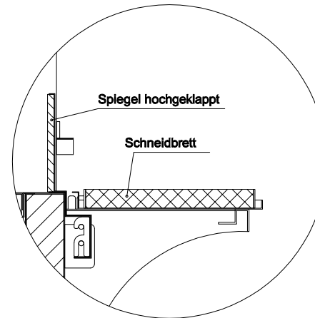
(Detail Spiegelsystem)
