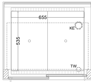
(Grundriss)
