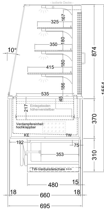
(Seitenansicht)
