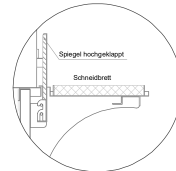
(Detail Spiegelsystem)
