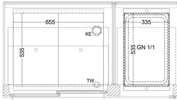
(Grundriss)
