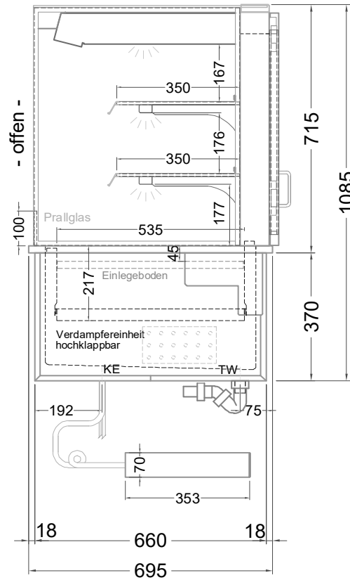
(Seitenansicht)
