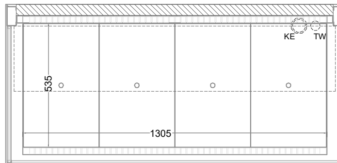
(Grundriss)
