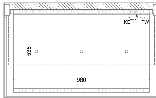
(Grundriss)
