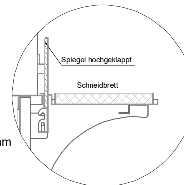
(Detail Spiegelsystem)
