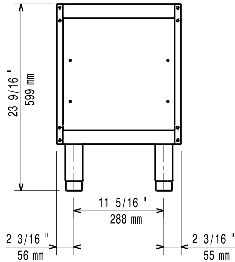
[Vorderansicht]
