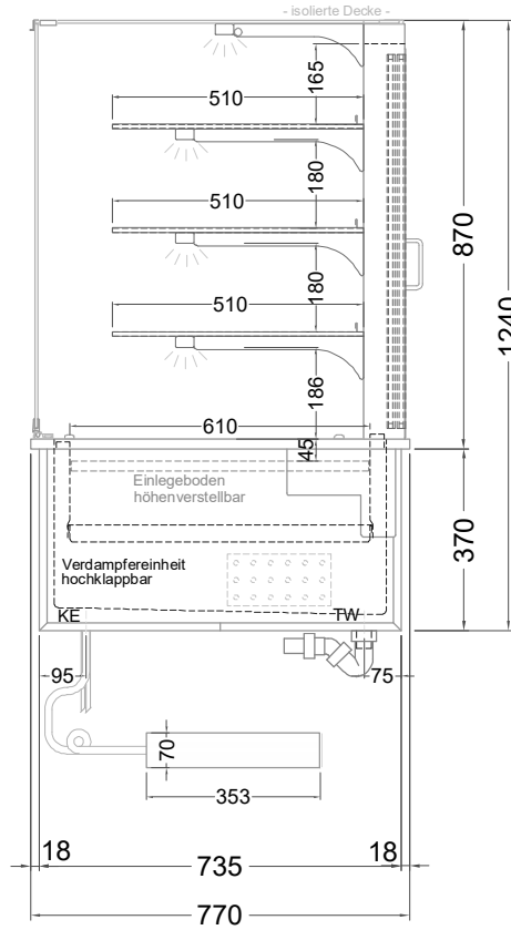
(Seitenansicht)
