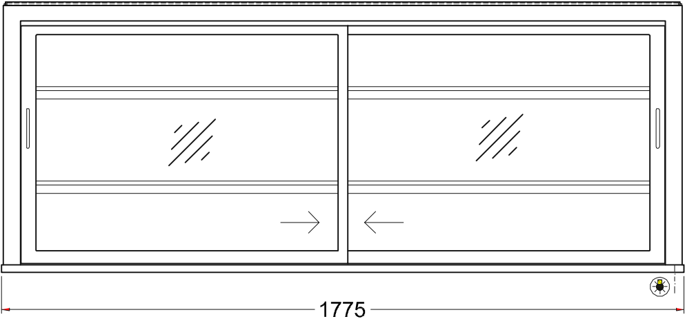
(Bedienseite)
