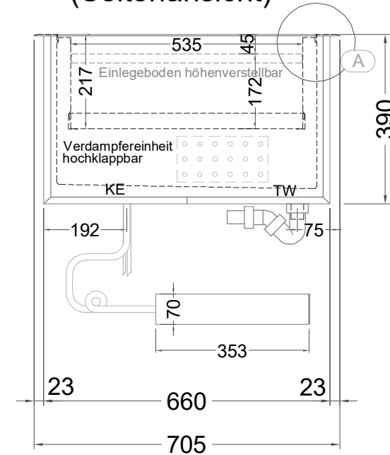
(Seitenansicht)
