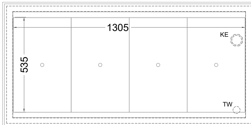
(Grundriss)
