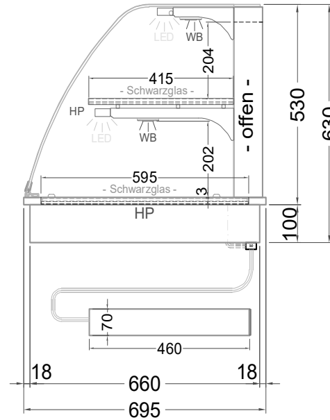
(Seitenansicht)
