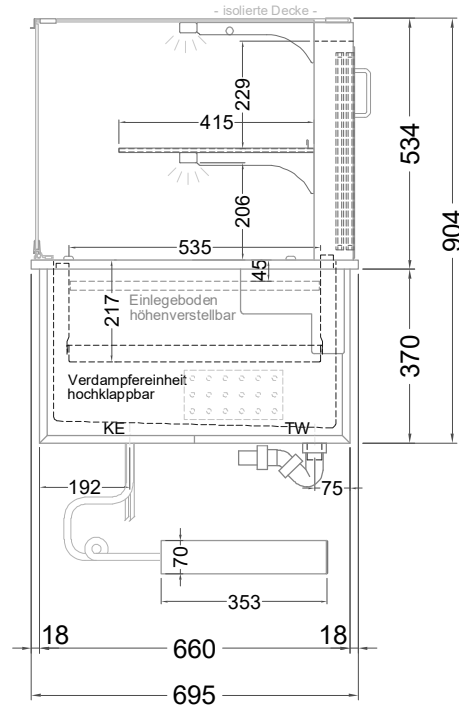
(Seitenansicht)
