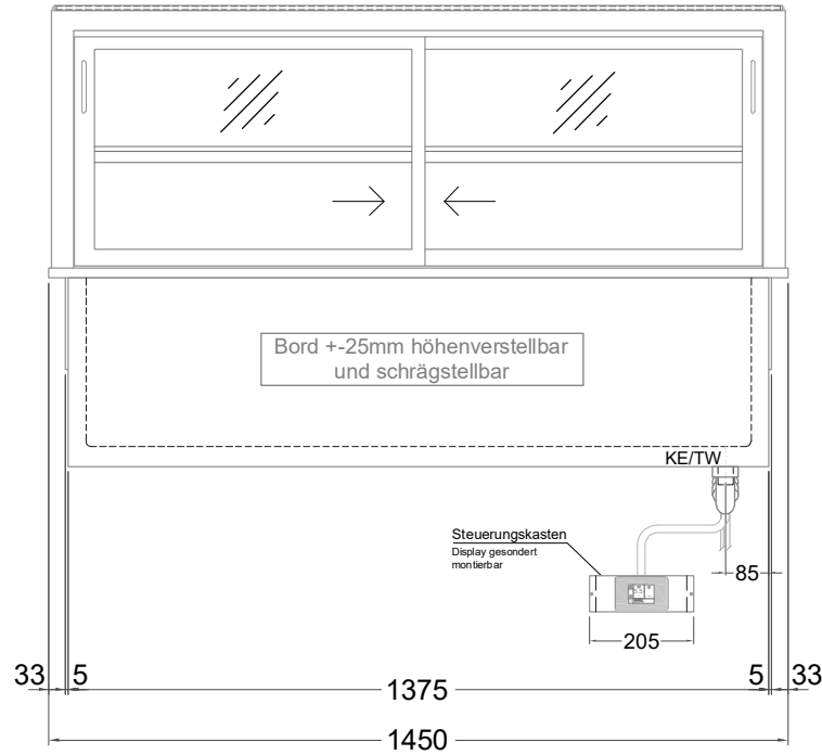
(Bedienseite)
