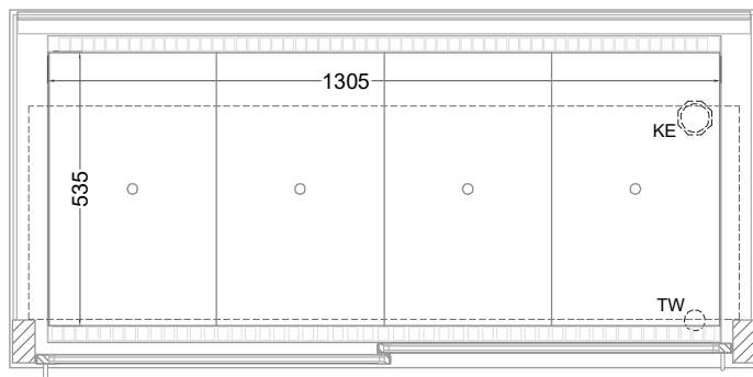
(Grundriss)
