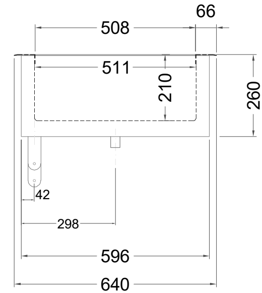
(Seitenansicht)
