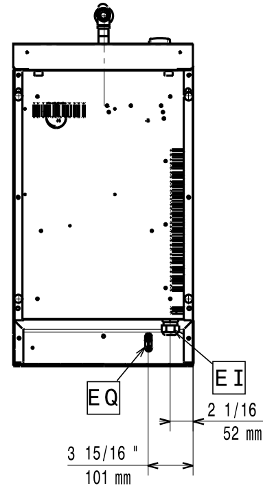
[Untersicht]
