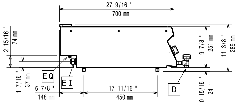
[Seitenansicht]
