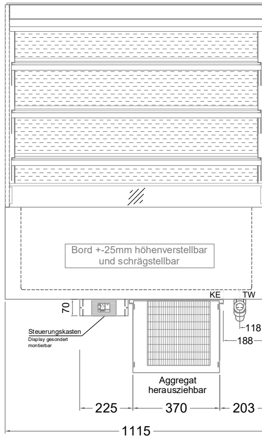
(Vorderseite)
