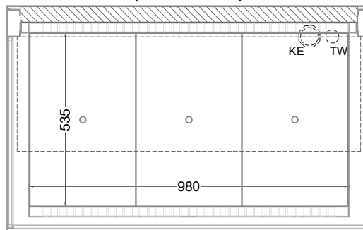
(Grundriss)
