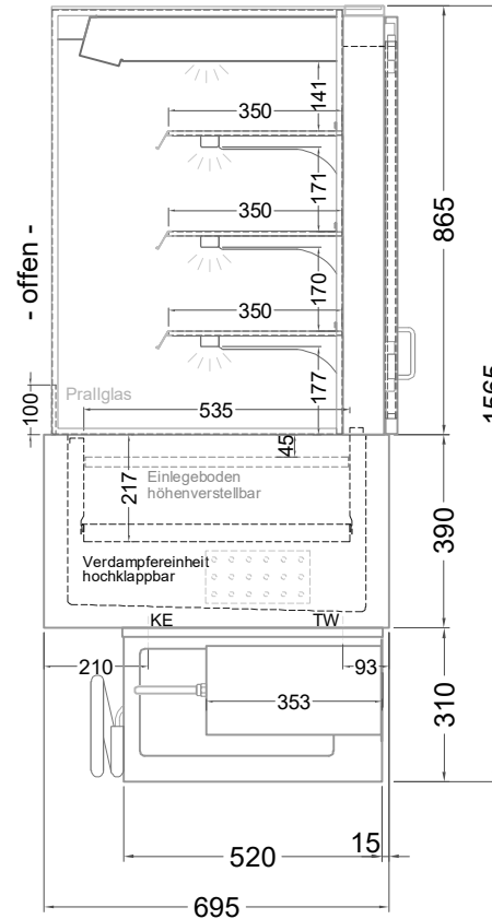
(Seitenansicht)
