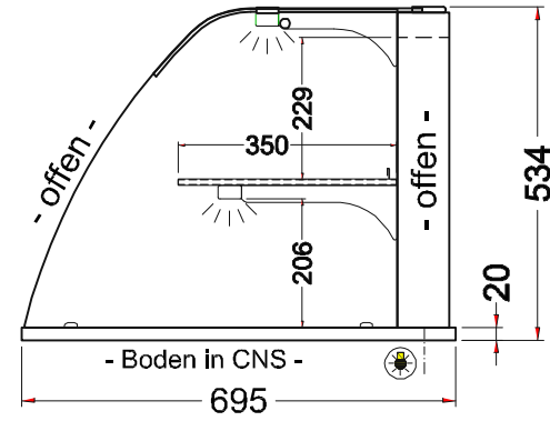
(Seitenansicht)
