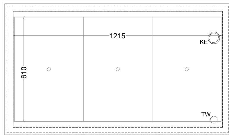
(Grundriss)
