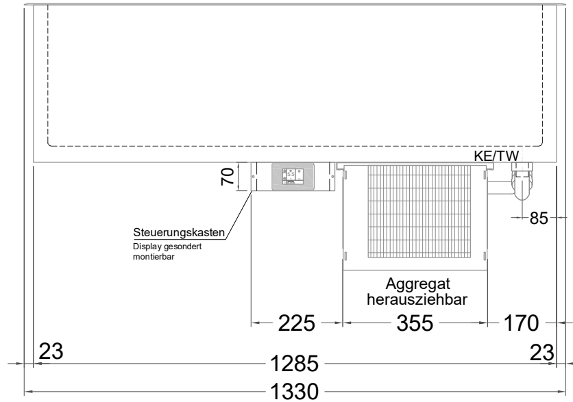
(Bedienseite)
