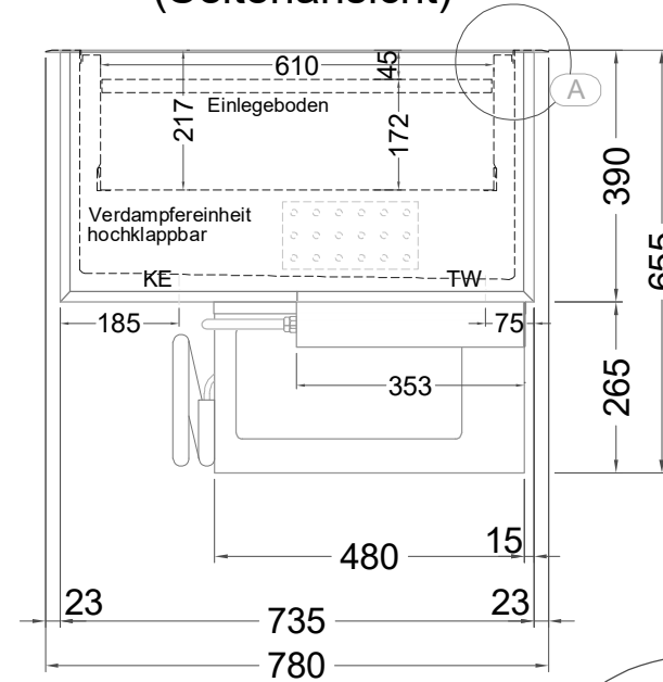
(Seitenansicht)
