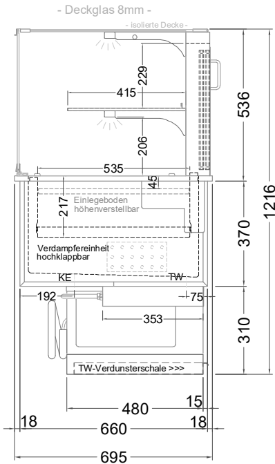
(Seitenansicht)
