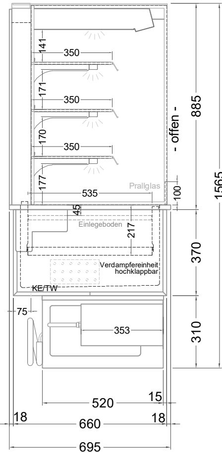
(Seitenansicht)
