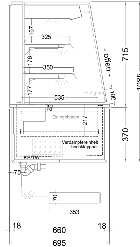
(Seitenansicht)
