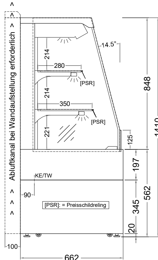
(Seitenansicht)
