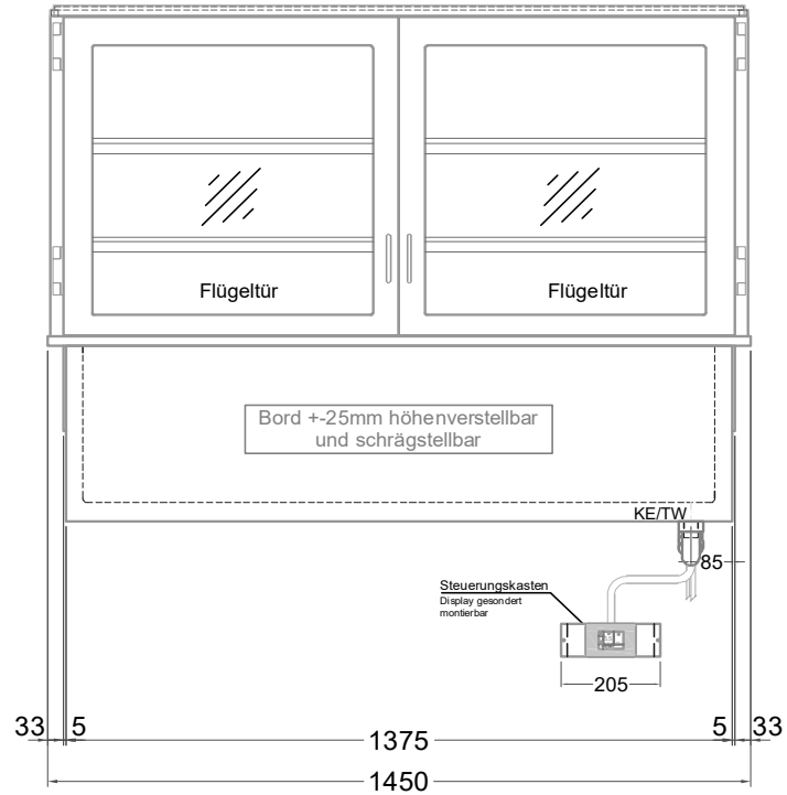
(Bedienseite)
