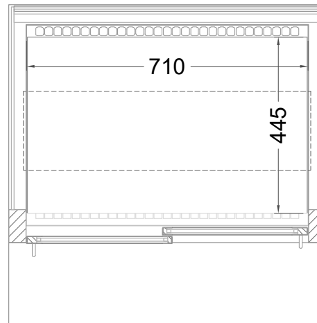
(Grundriss)
