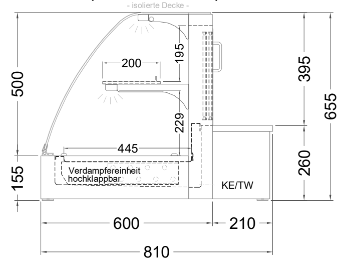
(Seitenansicht)
