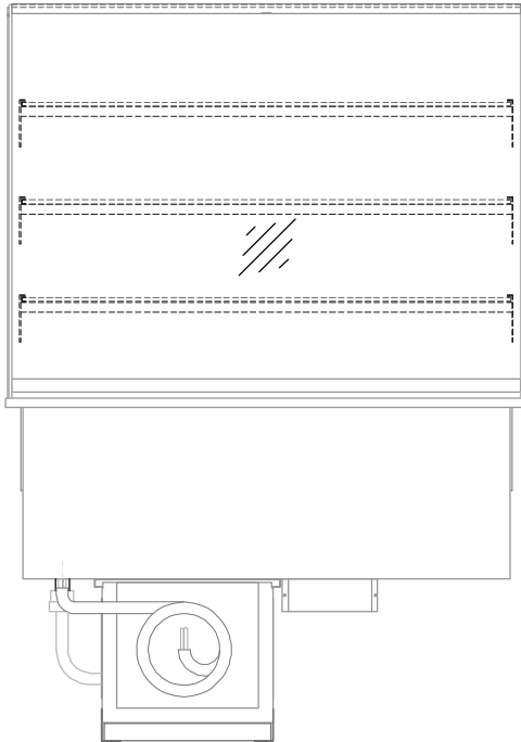
(Kundenseite)
