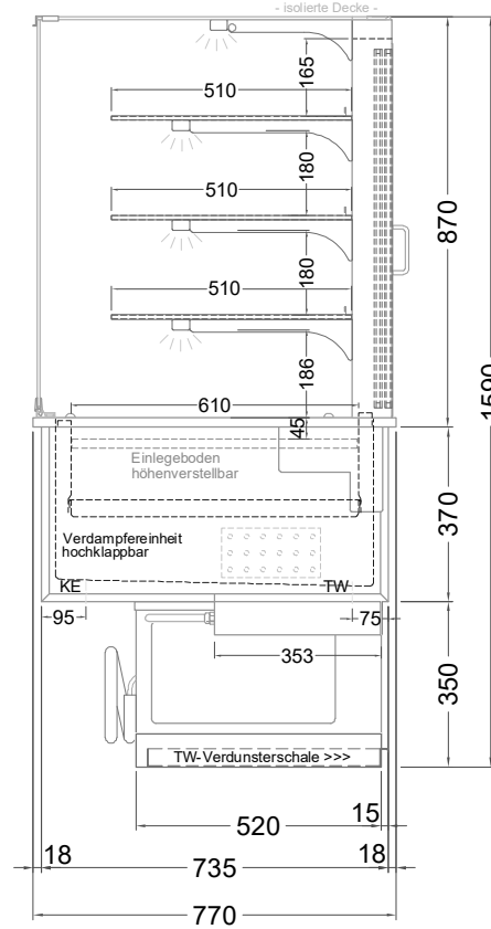
(Seitenansicht)
