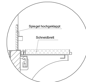
(Detail Spiegelsystem)
