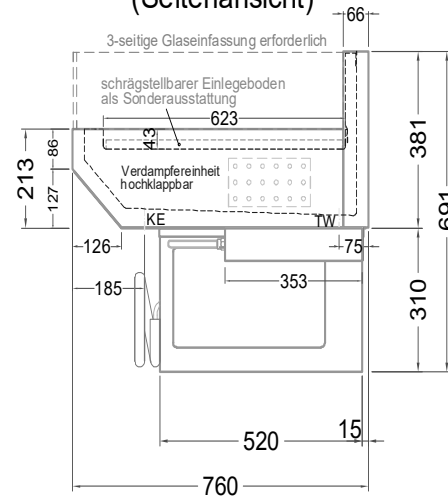
(Seitenansicht)
