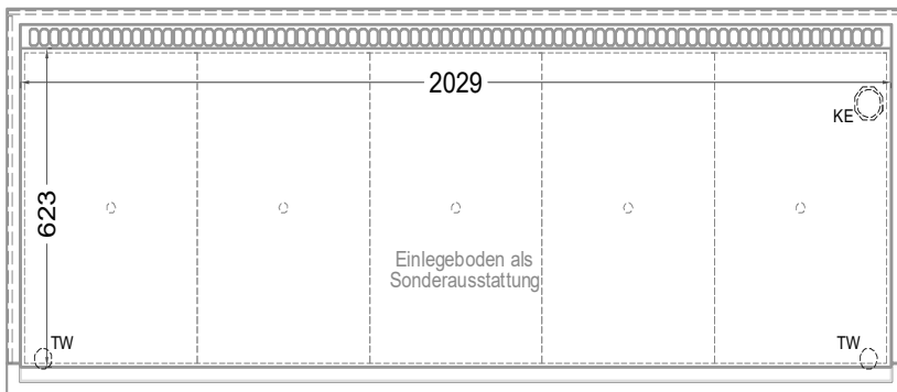
(Grundriss)
