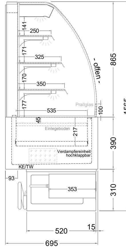
(Seitenansicht)
