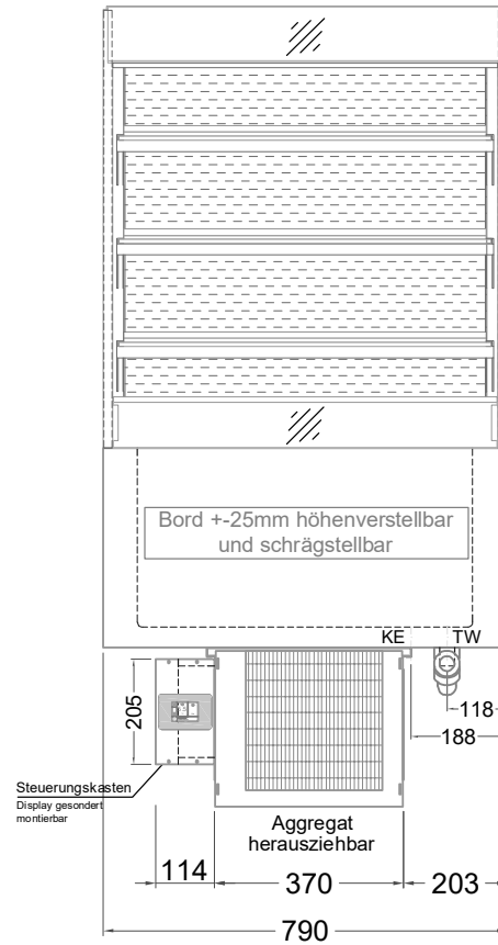
(Vorderseite)
