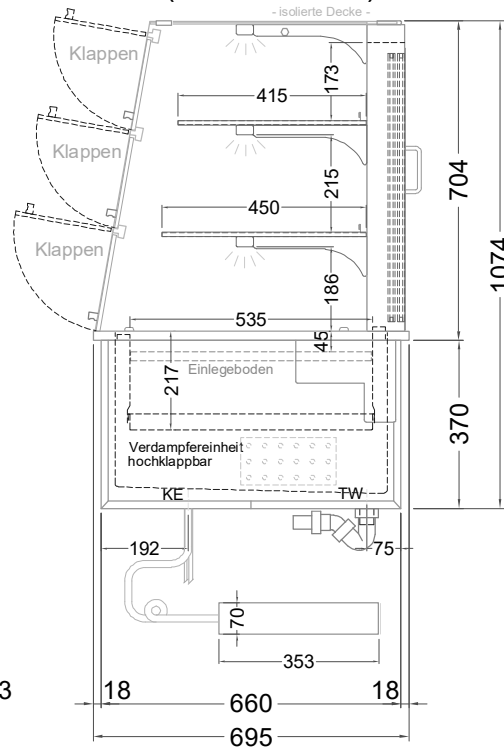
(Seitenansicht)
