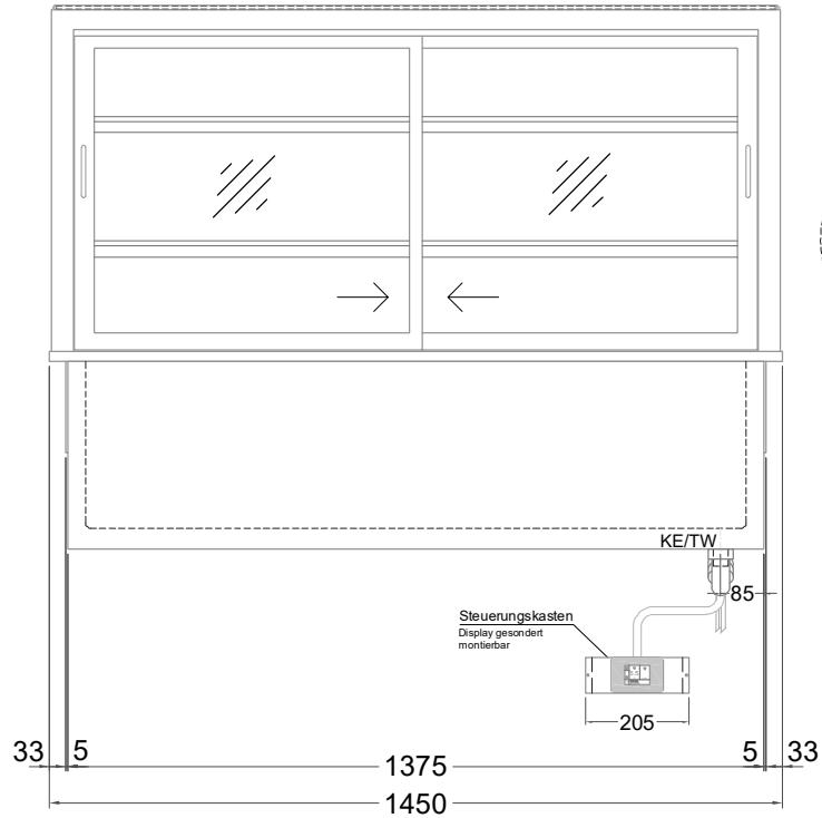
(Bedienseite)
