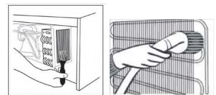
Abbildung 14: Kondensator reinigen
