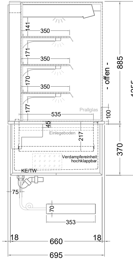
(Seitenansicht)
