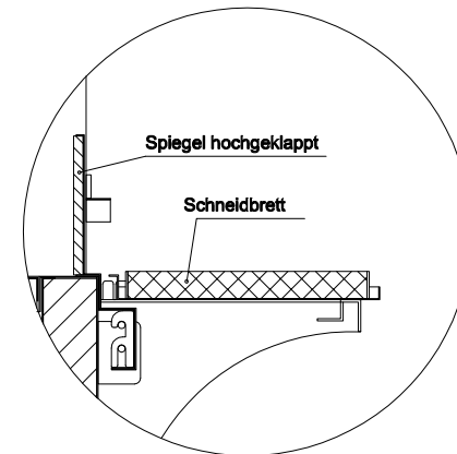
(Detail Spiegelsystem)
