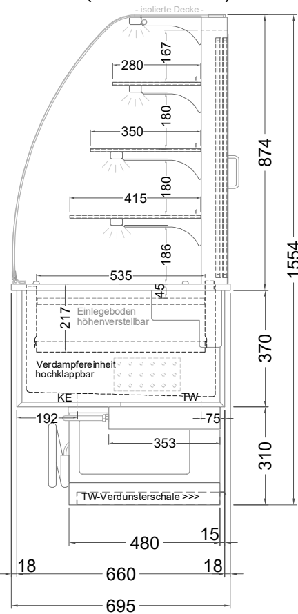
(Seitenansicht)
