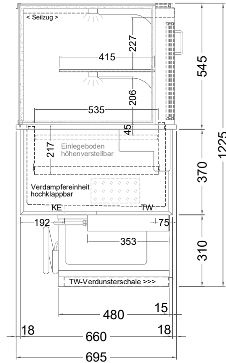
(Seitenansicht)
