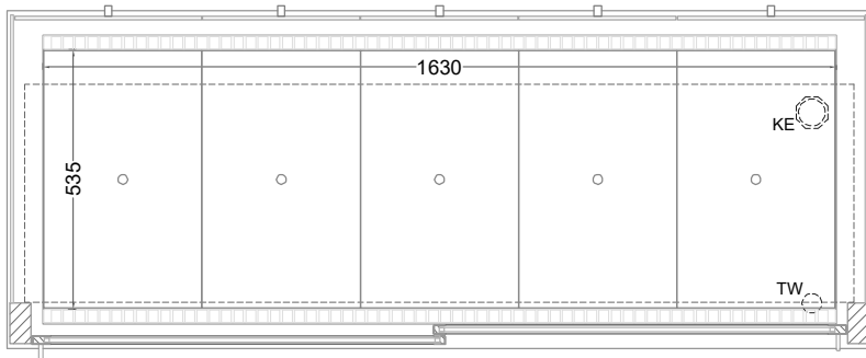
(Grundriss)
