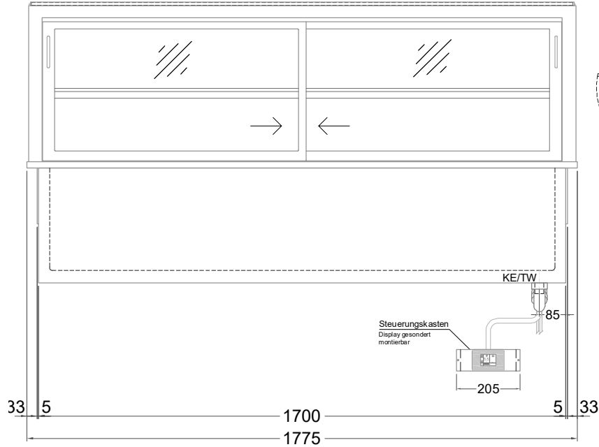
(Bedienseite)
