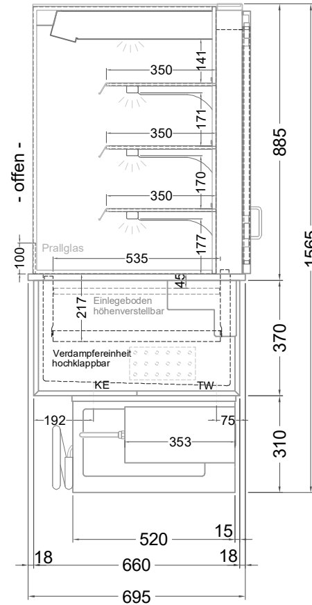
(Seitenansicht)
