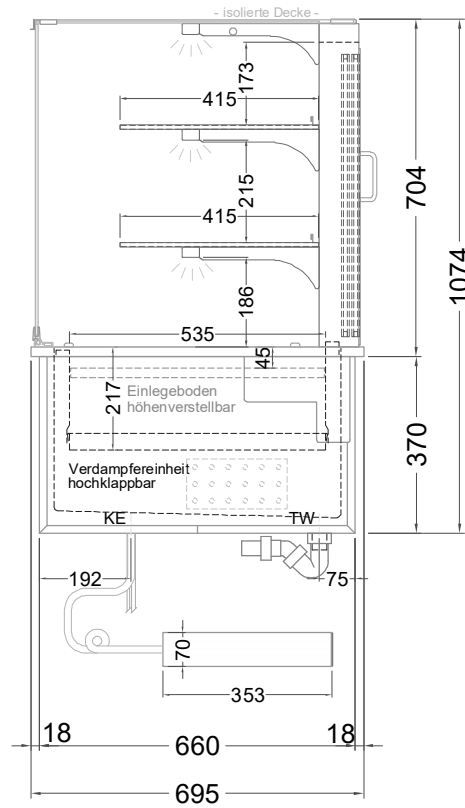
(Seitenansicht)
