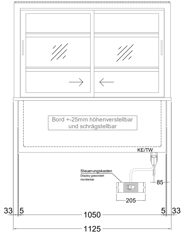
(Bedienseite)
