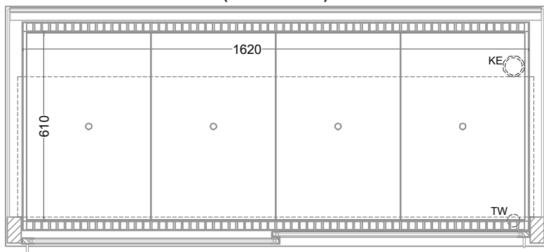
(Grundriss)
