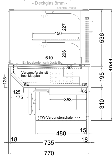
(Seitenansicht)
