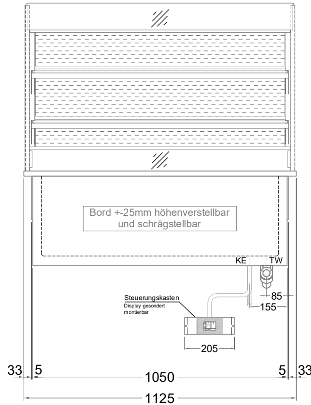
(Vorderseite)
