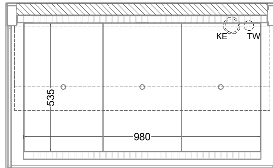
(Grundriss)
