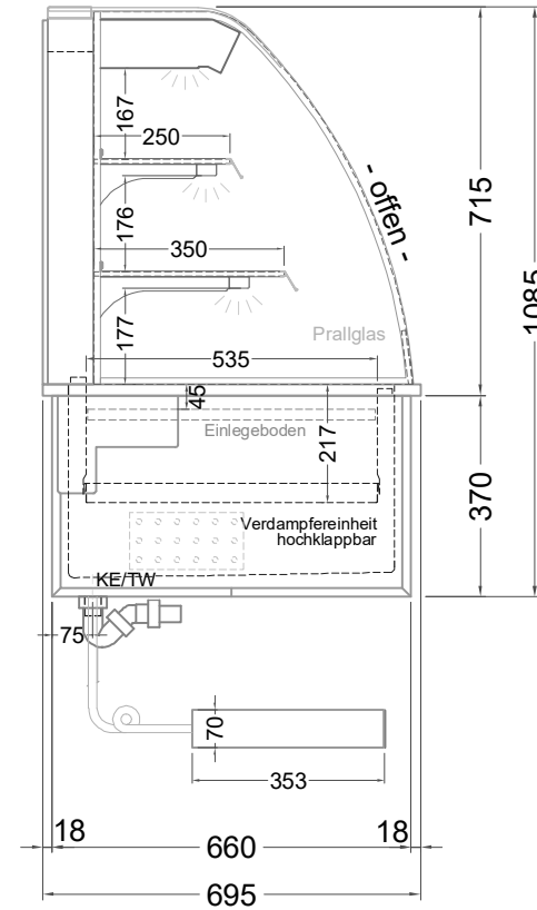
(Seitenansicht)
