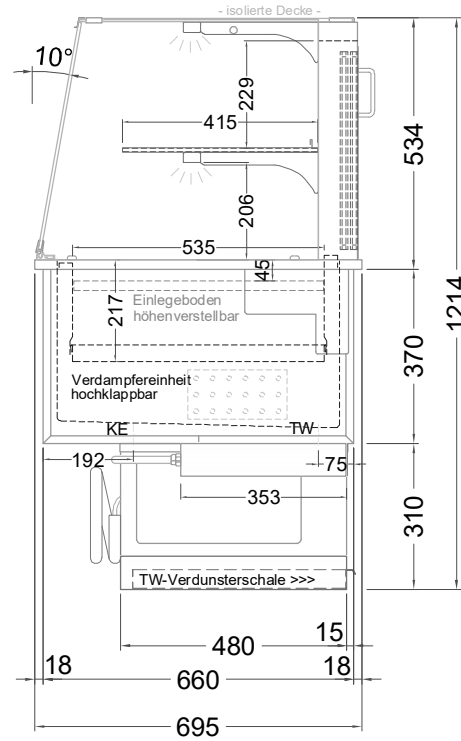
(Seitenansicht)
