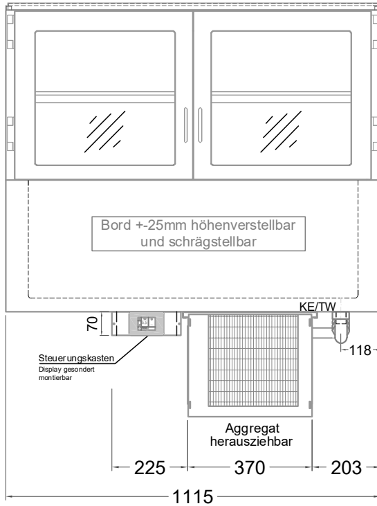
(Bedienseite)
