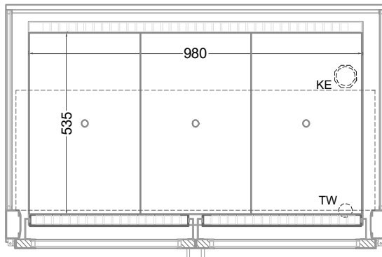
(Grundriss)
