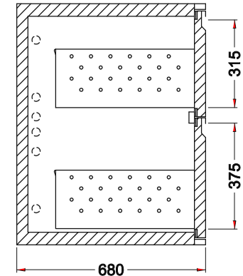
Schnitt L1
