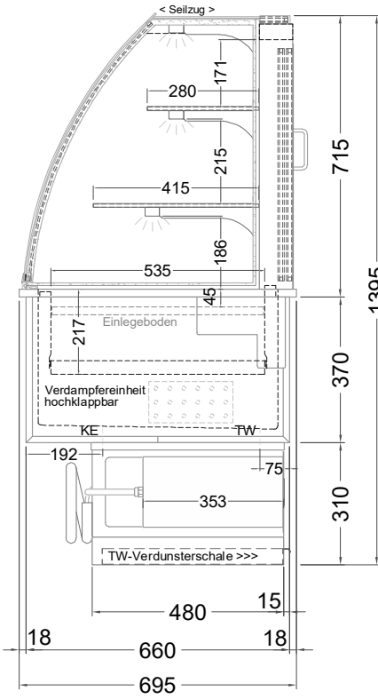
(Seitenansicht)
