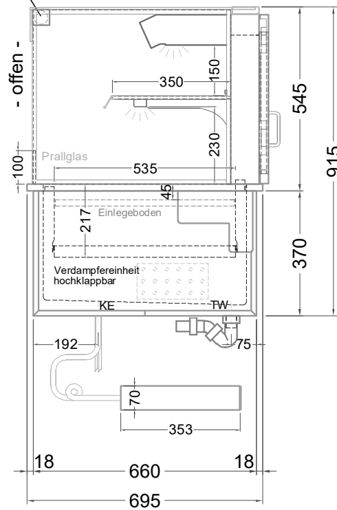
Rollo (Seitenansicht)
