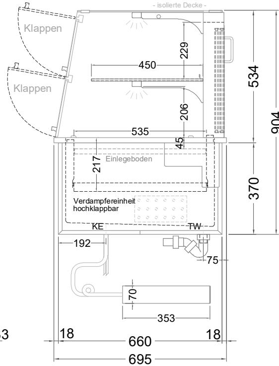
(Seitenansicht)
