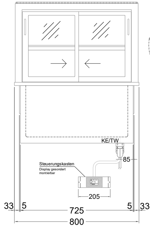
(Bedienseite)
