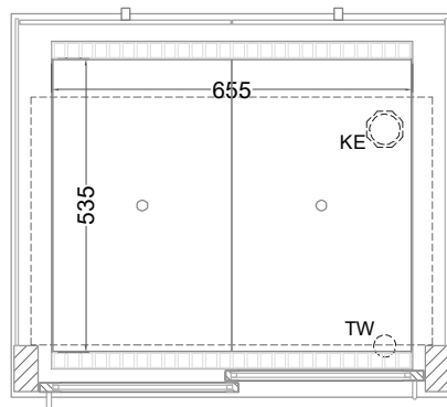
(Grundriss)
