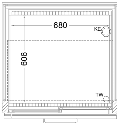
(Grundriss)
