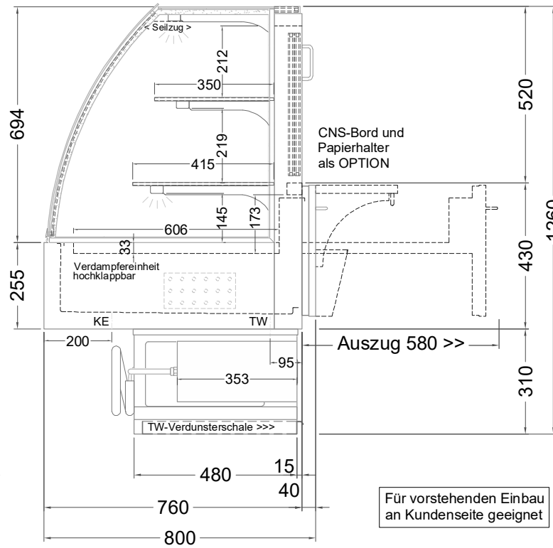
(Seitenansicht)
