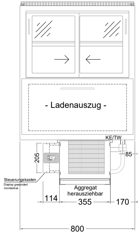
(Grundriss)
