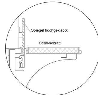
(Detail Spiegelsystem)
