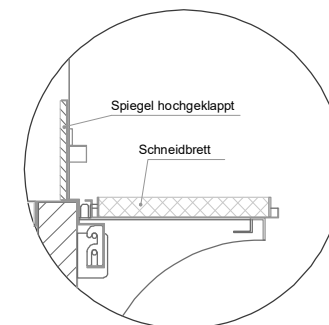
(Detail Spiegelsystem)
